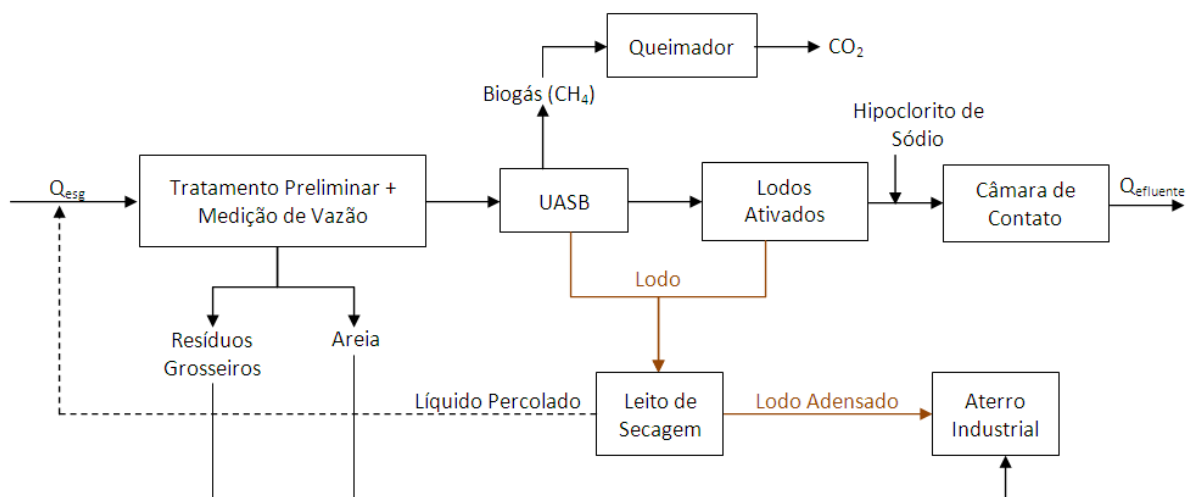
Figura 4.2 - Fluxograma do Sistema de Tratamento Previsto para o Bairro Paraíso
