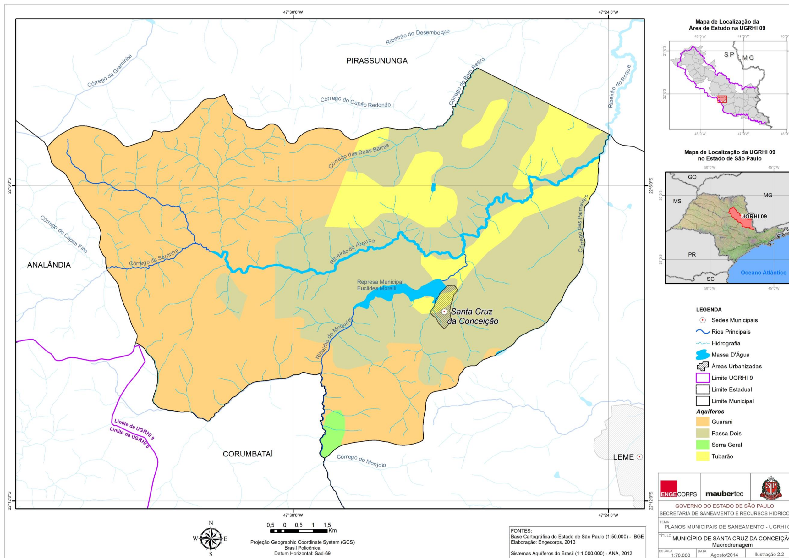
Ilustração 2.2 - Macrodrenagem
