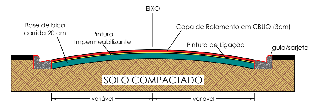
SEÇÃO TRANSVERSAL GERAL sem escala
